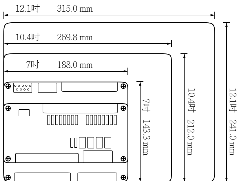
外觀尺寸圖
